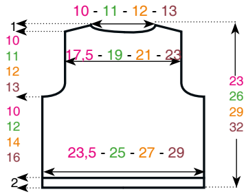
Patron dos
